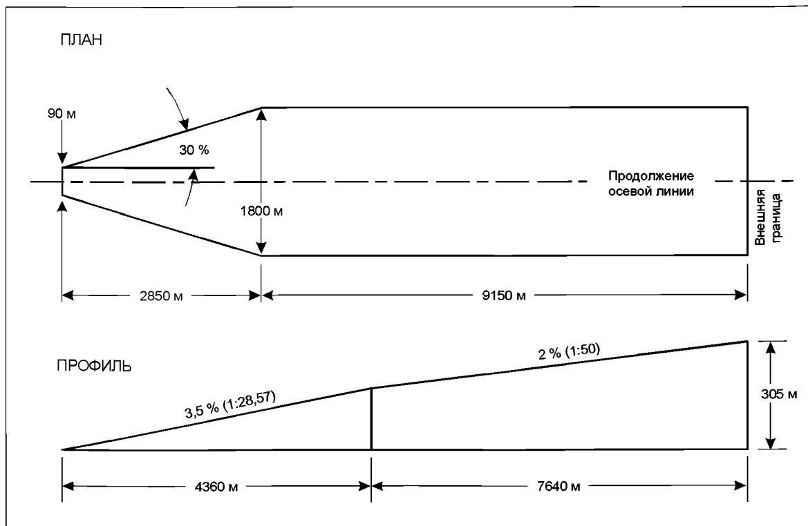
Рис. А2-2. Поверхность набора высоты при взлете для оборудованной FATO
